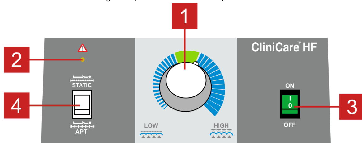
Fig. 13 Panneau de commande de l'unité SCU - CliniCare 100 HF sans le mode MCM
