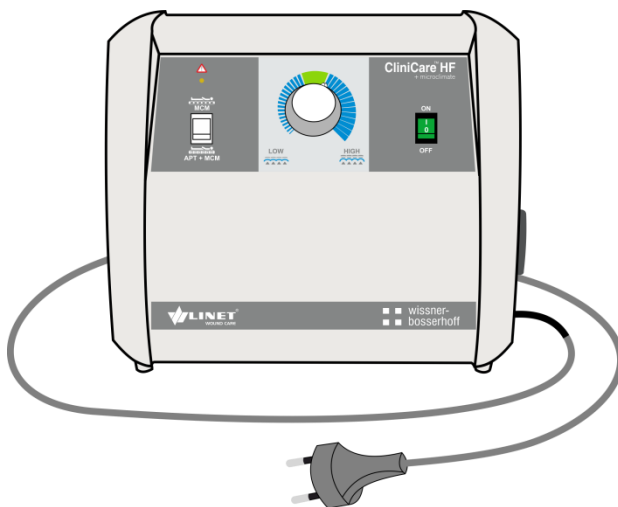
Fig. 3 Unité SCU pour CliniCare 100 HF avec le mode MCM
