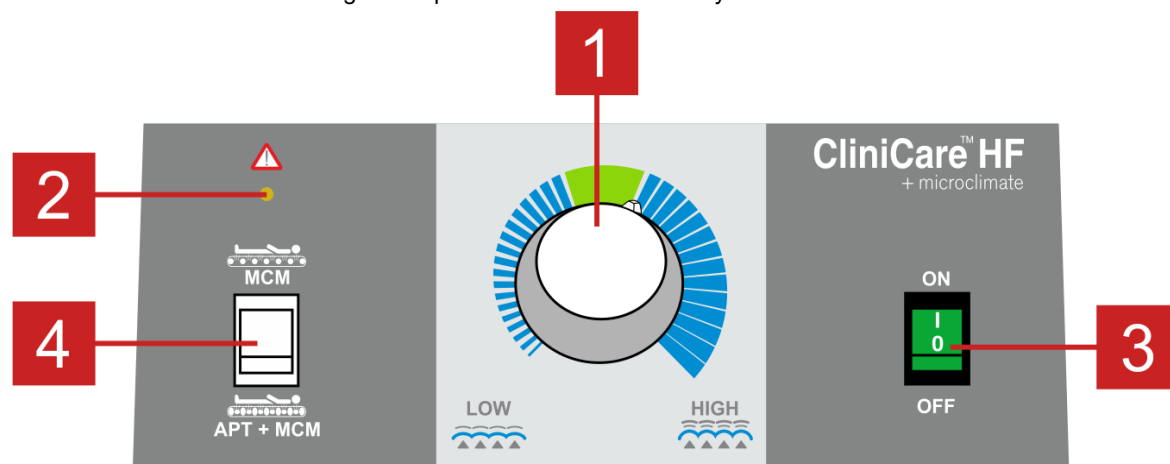
Fig. 12 Panneau de commande de l'unité SCU - CliniCare 100 HF avec le mode MCM
