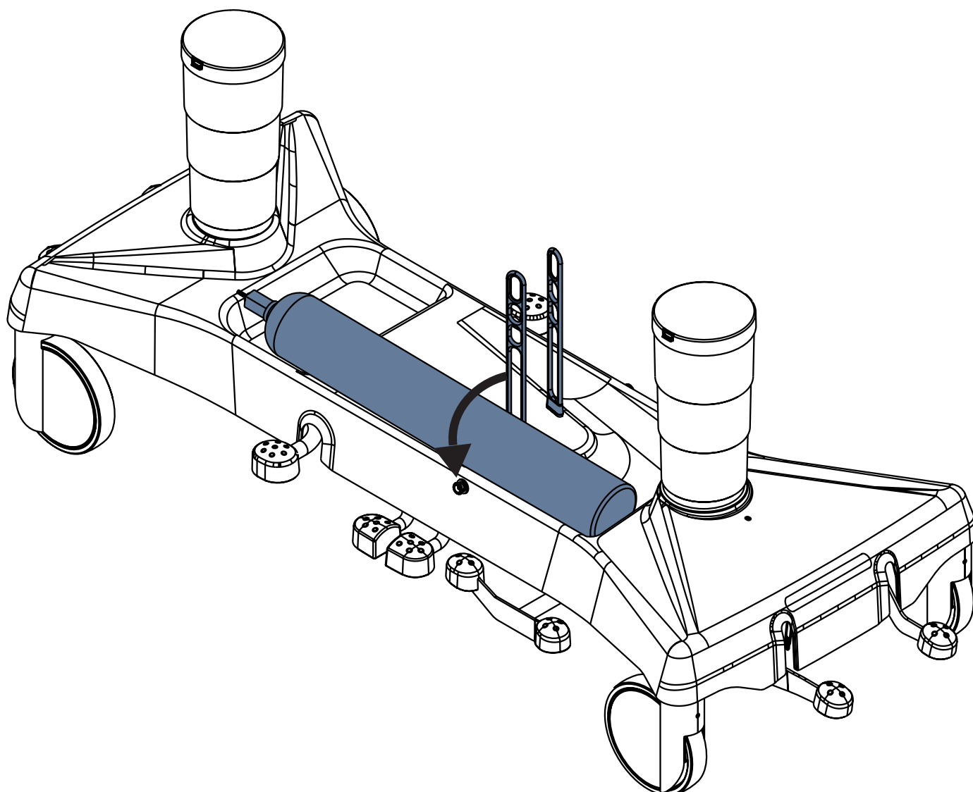
Fig. Fijación de una botella de oxígeno en la funda del bastidor con sujeciones para botellas de oxígeno
