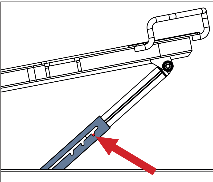
Fig. Detalle de la posición de enganche en la barra de trinquete
