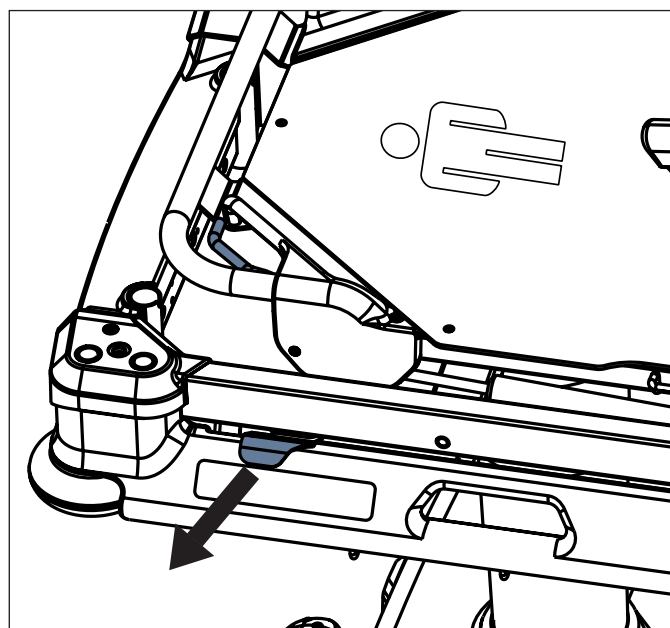
Fig. Manipulación con mecanismo de liberación de la barandilla del cabecero
