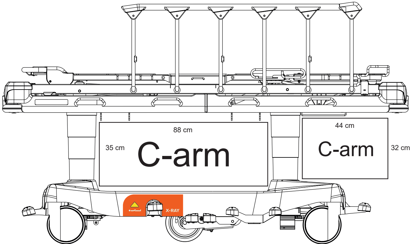
Fig. Espacio para la parte inferior de un brazo en C
