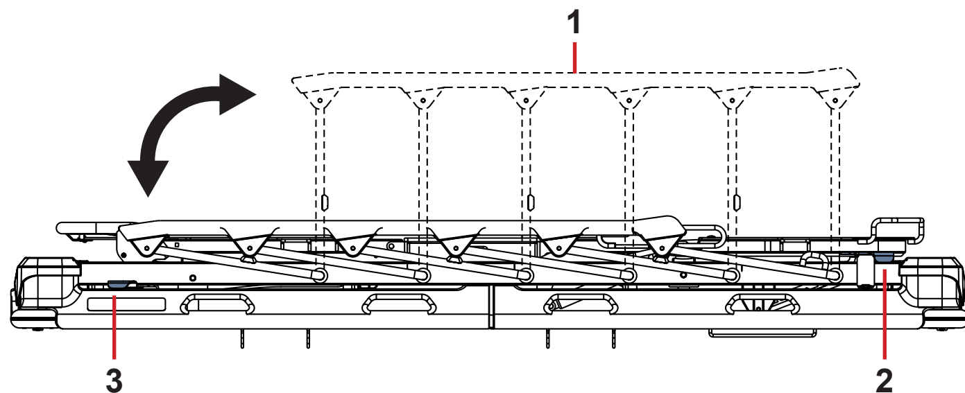
Fig. Manipulación con barandilla plegable
