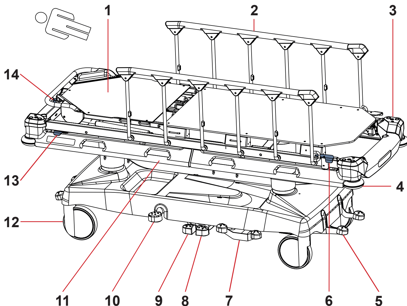
Fig. Resumen de la cama (Sprint 100 con plataforma de apoyo del colchón de 2 partes)
