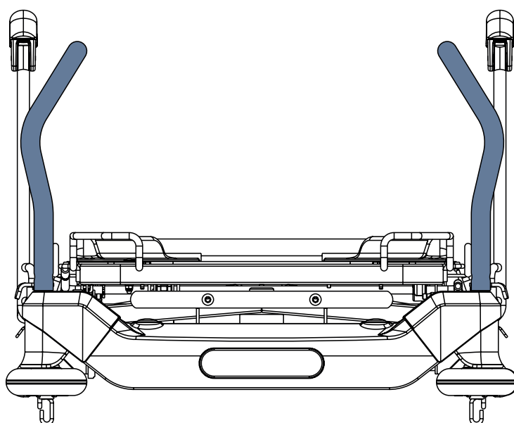
Fig. Asas extraíbles (vista frontal)
