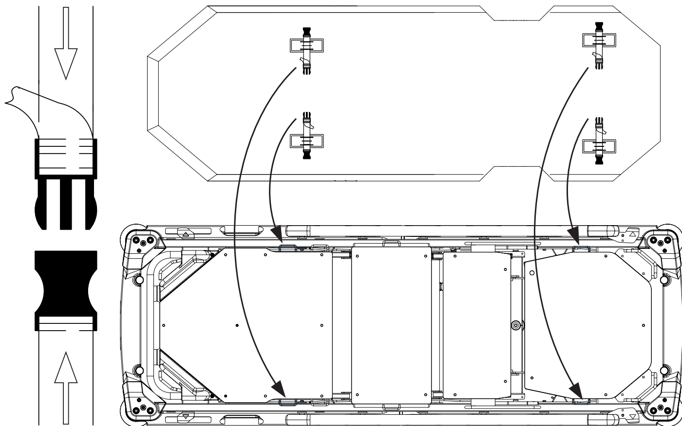
Fig. Fijación del colchón con cintas en la Sprint 100 con plataforma de apoyo del colchón de 4 piezas
