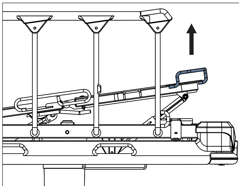
Fig. Colocación del reposapiés
