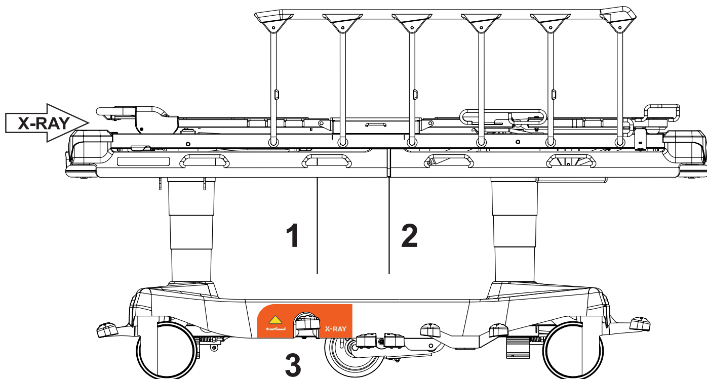
Fig. Sprint 100 con plataforma de apoyo del colchón de 4 piezas (equipada con soporte para chasis radiográfico)
