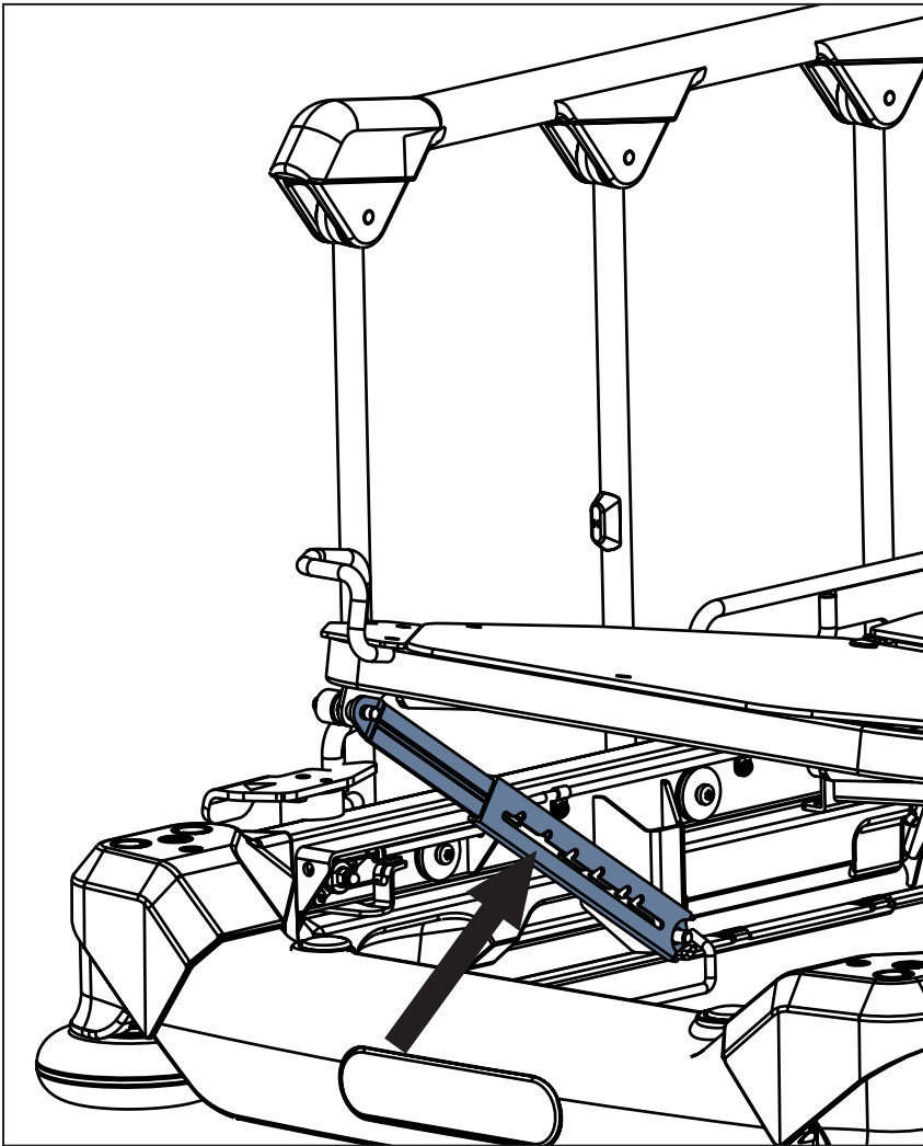
Fig. Barra de trinquete del reposapiés
